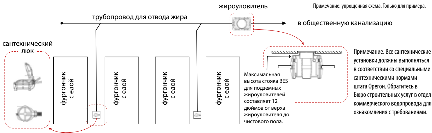
Рисунок группы фургончиков с едой с надлежащим подсоединением к бытовой канализации
