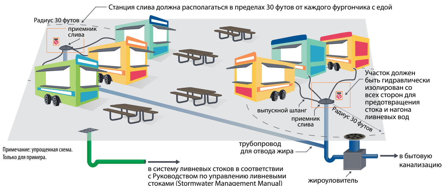
Рисунок группы фургончиков с едой с надлежащим подсоединением к бытовой канализации
